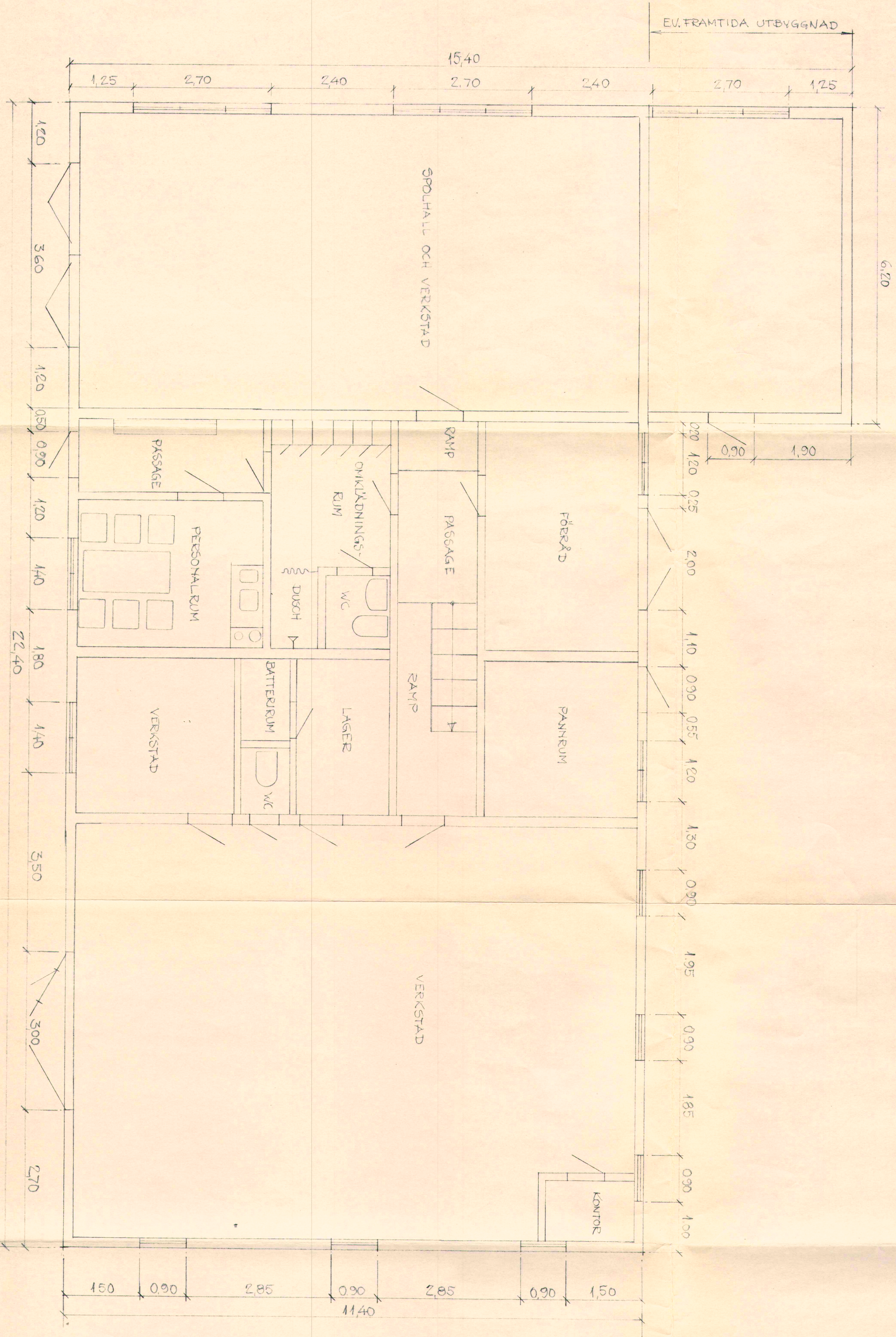
PLAN.
